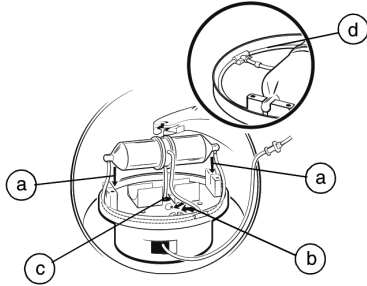
Şekil 3. Ayırma bölmesini taşıyıcıya kurun ve tüpü yuva içine ve tutucu altına yerleştirin.
