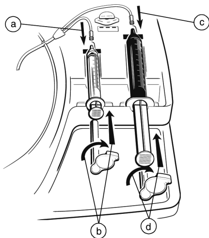
Figure 7. Monter la tubulure, charger les seringues et mettre en prise les dispositifs d'entraînement de piston de seringue.
