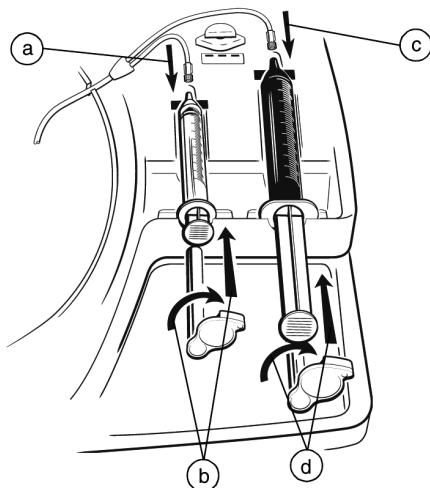
Figura 7. Collegare il tubo, caricare le siringhe e innestare gli azionatori degli stantuffi delle siringhe.
