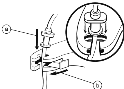
Figur 4. Anslut kammarens slangkrage till instrumentets stödarm för slangen.
