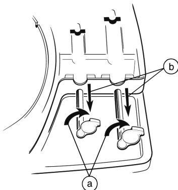
Afbeelding 6. In de spuithouders de open zuigermeenemers naar het laagste punt schuiven.
