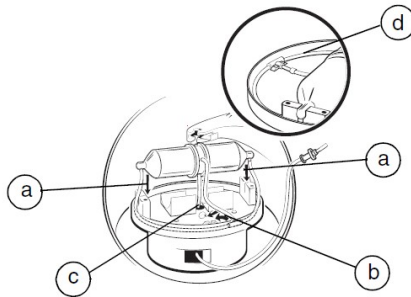
Εικόνα 9. Εγκαταστήστε τον θάλαμο διαχωρισμού στη θήκη και τοποθετήστε τη σωλήνωση μέσα στη σχισμή και κάτω από τη διάταξη συγκράτησης.
