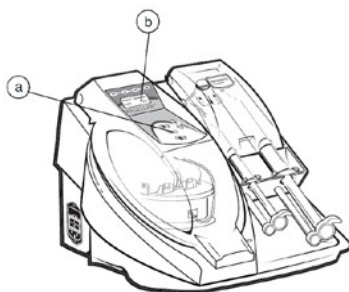
Figur 2. Arterioocyte Medical Systems MAGELLAN® instrumentet til separation af autologe trombocytter set forfra.
